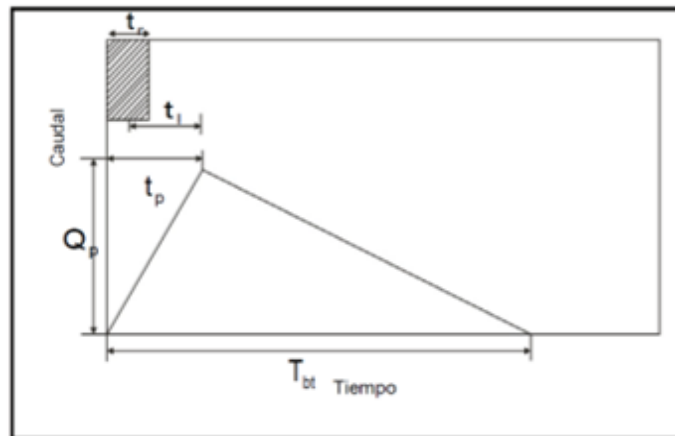
Figura 24. Hidrograma Unitario Triangular del SCS Fuente: (Chow, Madiment, & Mays, 1994).
