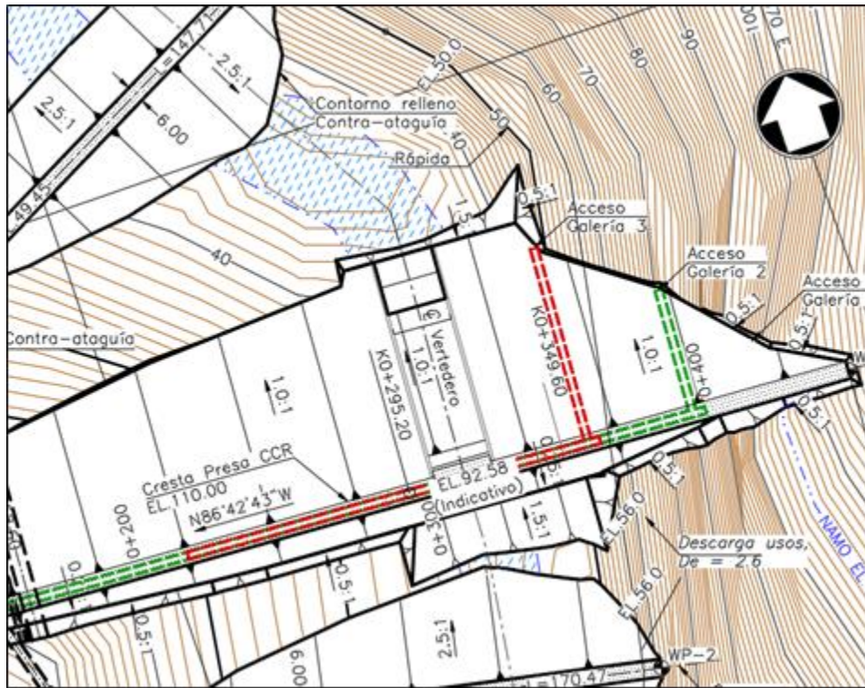
Figura 49. Planta General Vertedero - Perales
