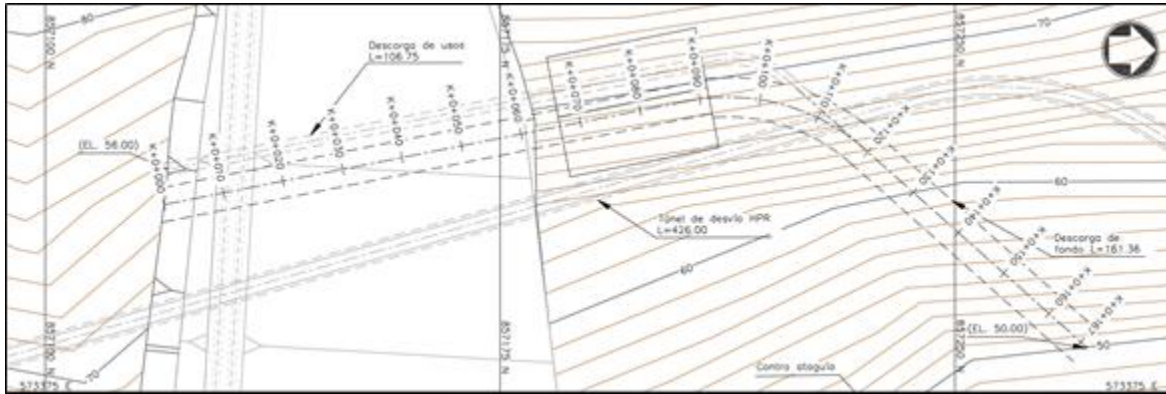
Figura 48. Esquema de la entrega de caudales de usos - Perales
