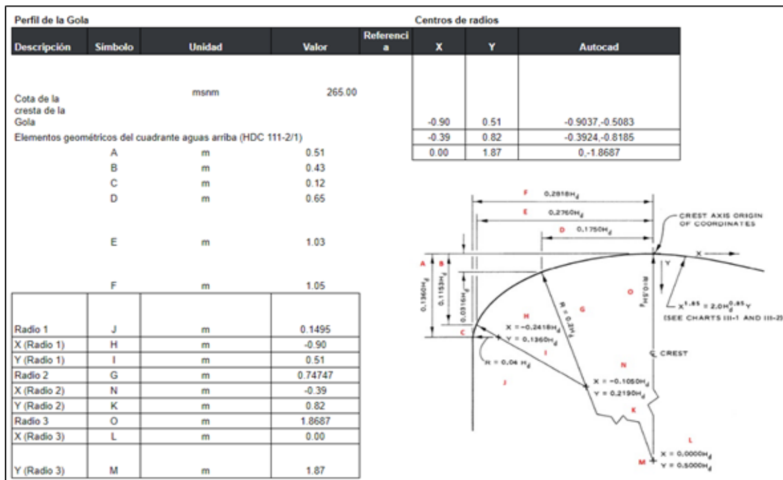
Figura 51. Perfil elíptico de la Gola en su parte trasera - Perales
