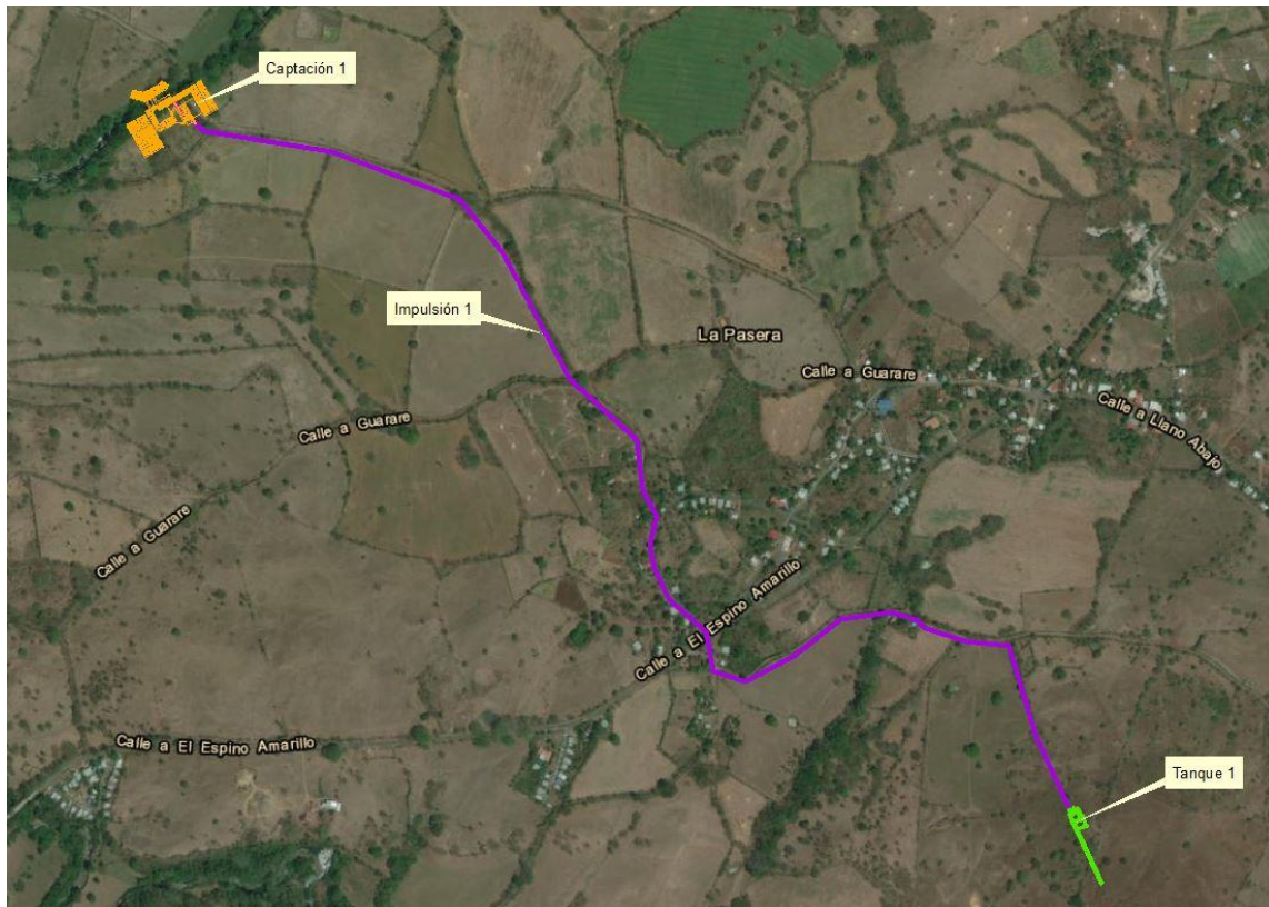
Figura 9. Infraestructura Existente Bombeo 1
