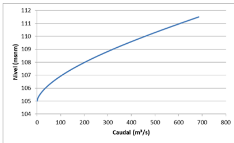
Figura 34. Curva de descarga vertedero Perales
