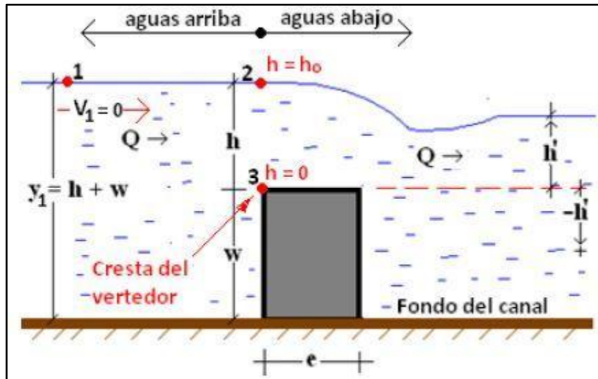
Figura 39. Parámetros Vertedero Rectangular de Pared Guesa
