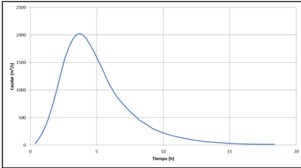
Figura 25. Hidrograma unitario sintético de la CMP - Perales
