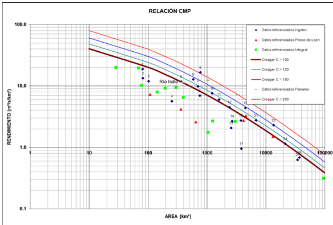
Figura 23. Envolvente de Creager
