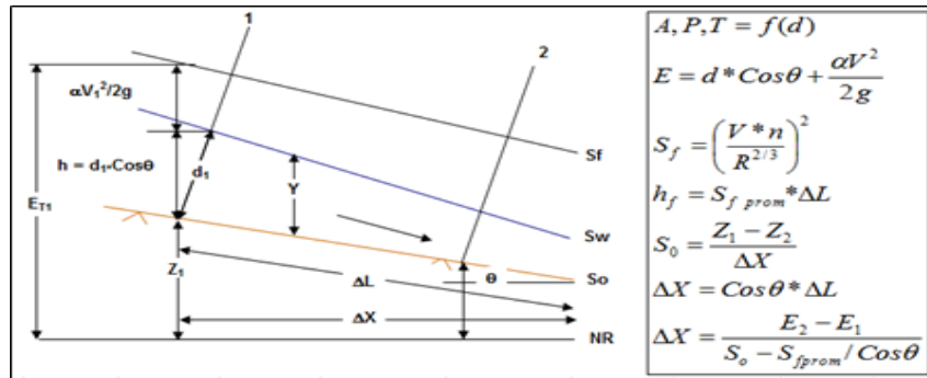
Figura 33. Ecuaciones básicas del flujo gradualmente variado
