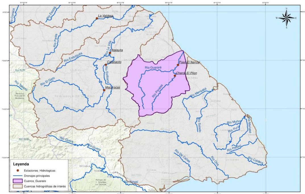
Figura 15. Cuenca del Río Guararé
