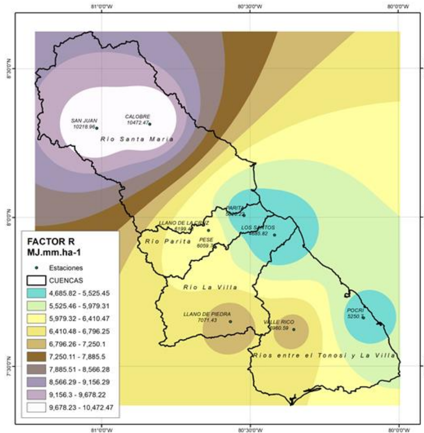
Figura 27. Distribución espacial del Factor R
