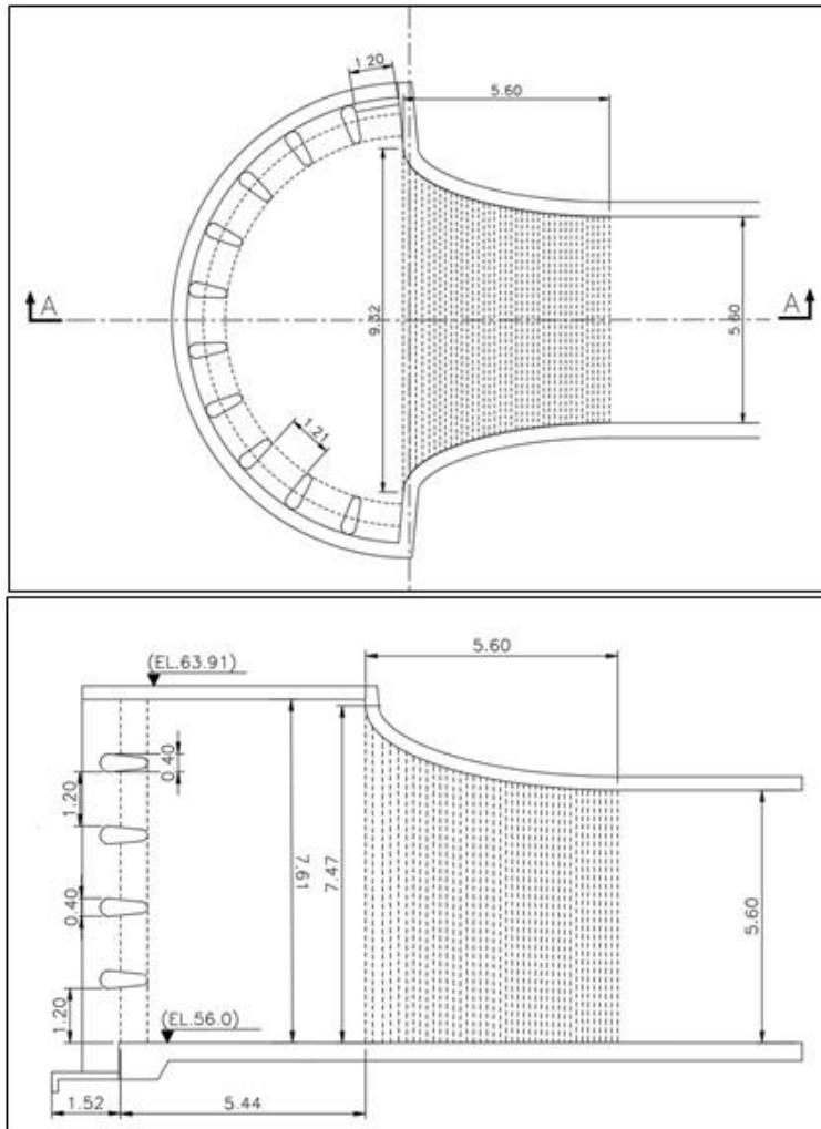
Figura 44. Esquema general de la captación de la descarga de fondo Perales
