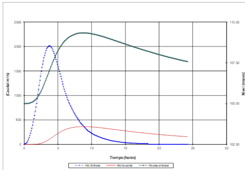
Figura 50. Curva de tránsito vertedero – Perales
