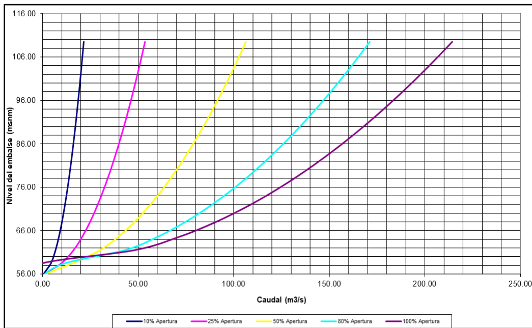
Figura 43. Capacidad hidráulica de la descarga de fondo
