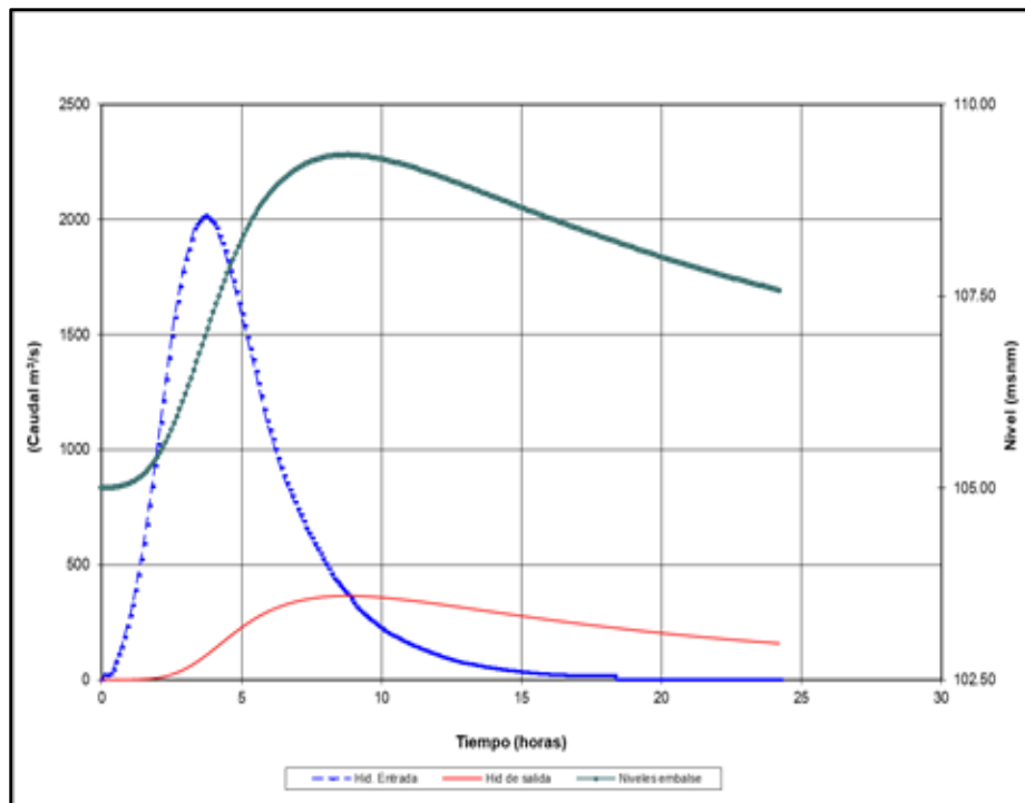
Figura 26. Tránsito del hidrograma de la CMP en el reservorio Perales
