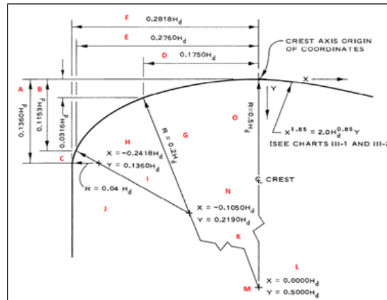
Figura 35. Parámetros Perfil Gola
