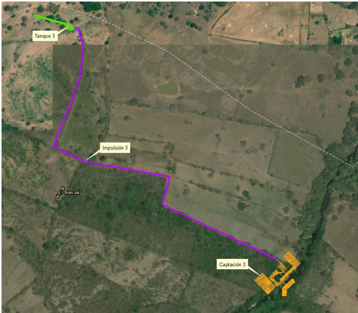
Figura 12. Infraestructura Existente Bombeo 3
