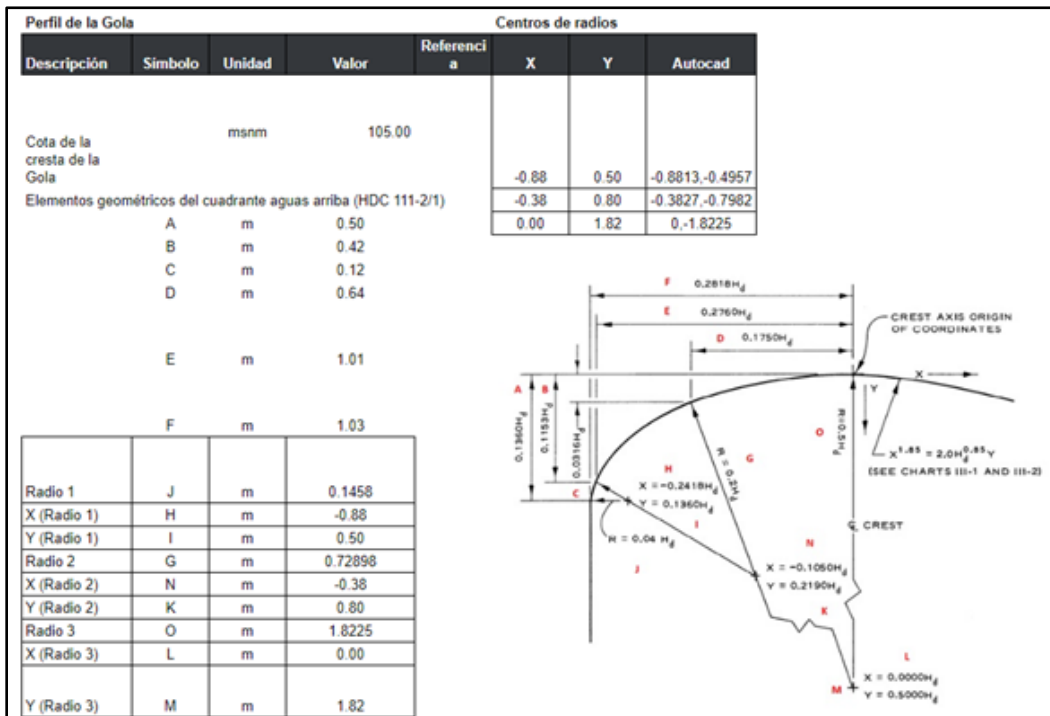
Figura 36. Parámetros Gola - Perales
