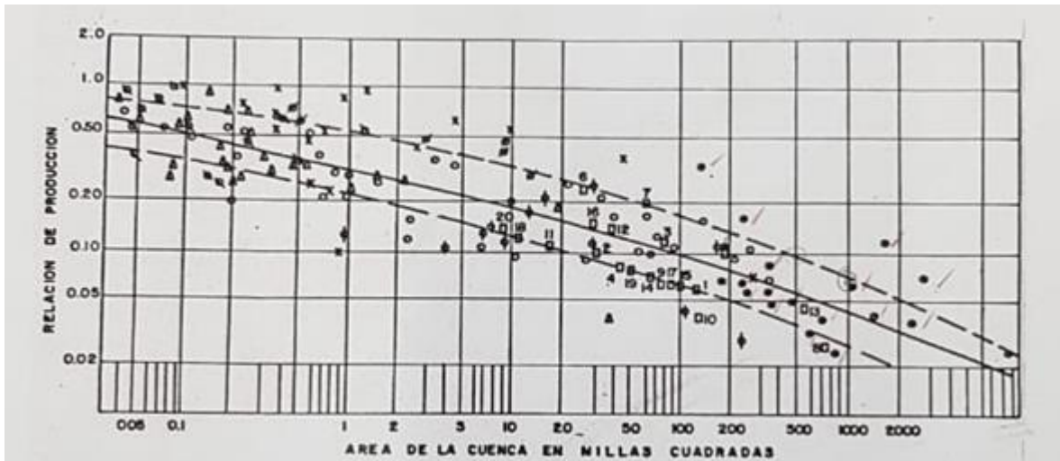
Figura 31. Relación de producción respecto al área de la cuenca (tomado del documento “Determinación de Coeficientes de Producción de Sedimentos en Cuencas Extensas”)
