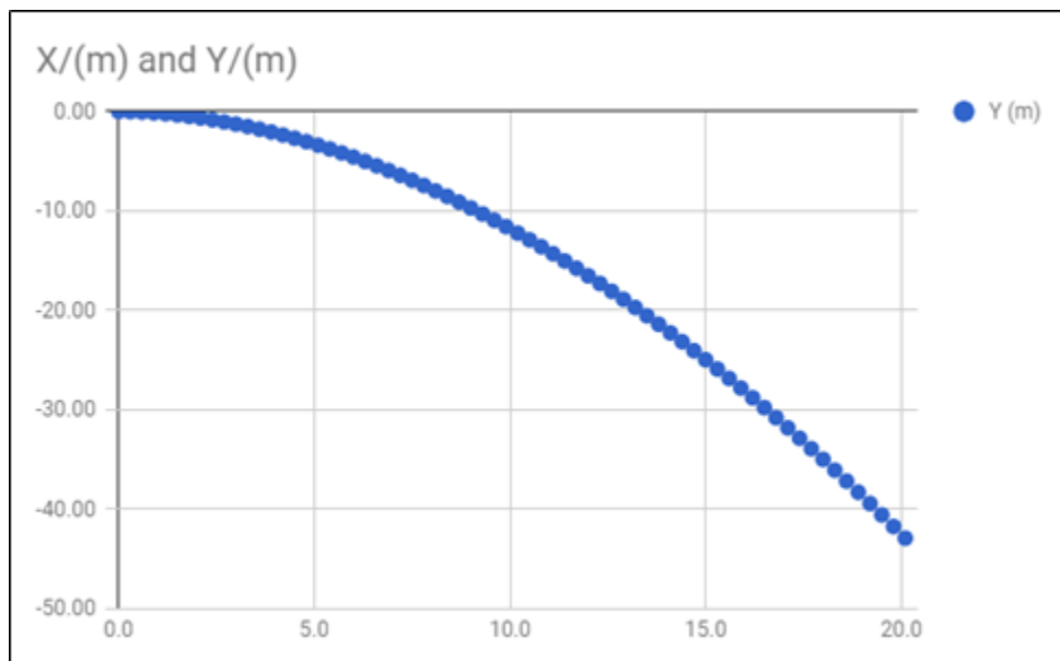
Figura 52. Perfil Gola – Perales
