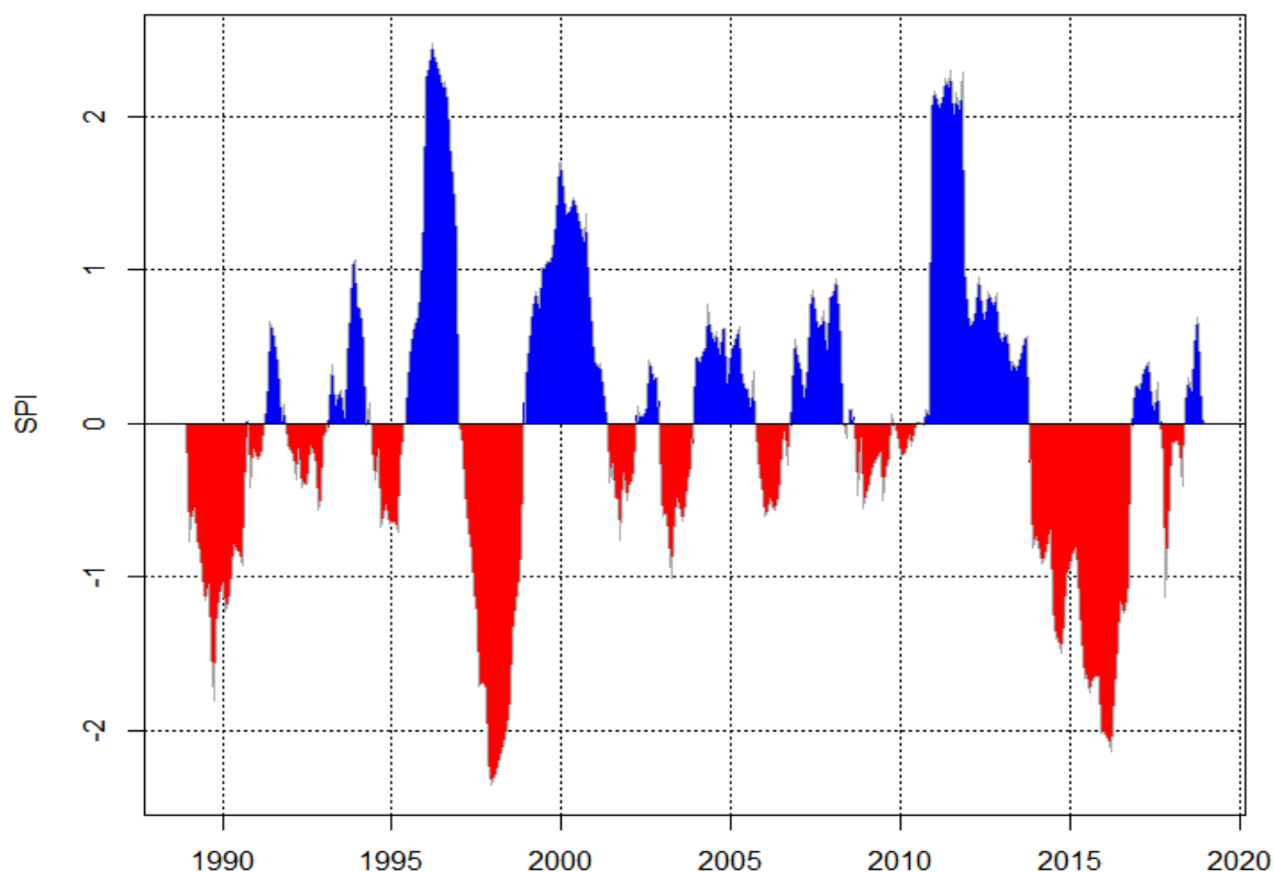
Figura 34. Evolución histórica del SPI en la CHCP (1988-2018)
