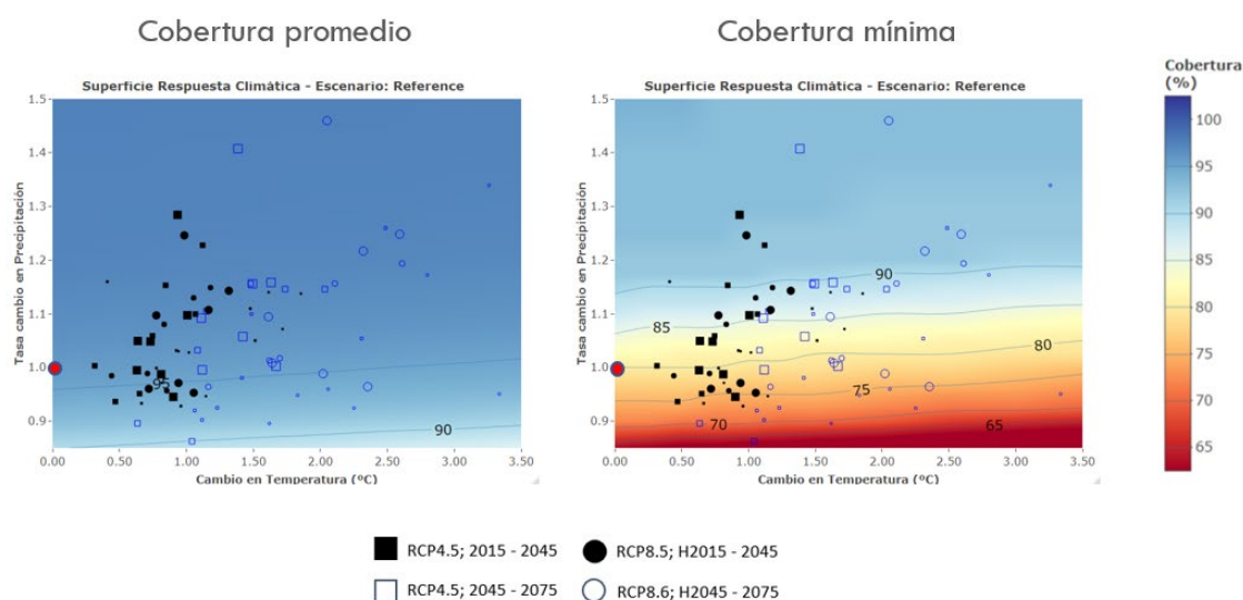
Figura 77. SRC para la condición de línea de base y la cobertura anual promedio de la Cuenca (panel izqdo.), y la cobertura mínima (panel dcho.). Los símbolos en negro y azul representan las tasas de cambio proyectadas por los diferentes modelos regionales del ensamble NEX-GDDP para diferentes trayectorias de emisión (RCP 4.5 y 8.5) y horizontes temporales (H2015-2045, H2045-2075).
