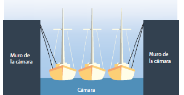
Vista frontal de los barcos amarrados
