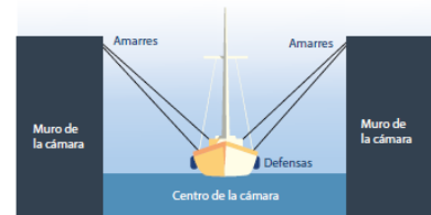
Vista frontal del barco amarrado
